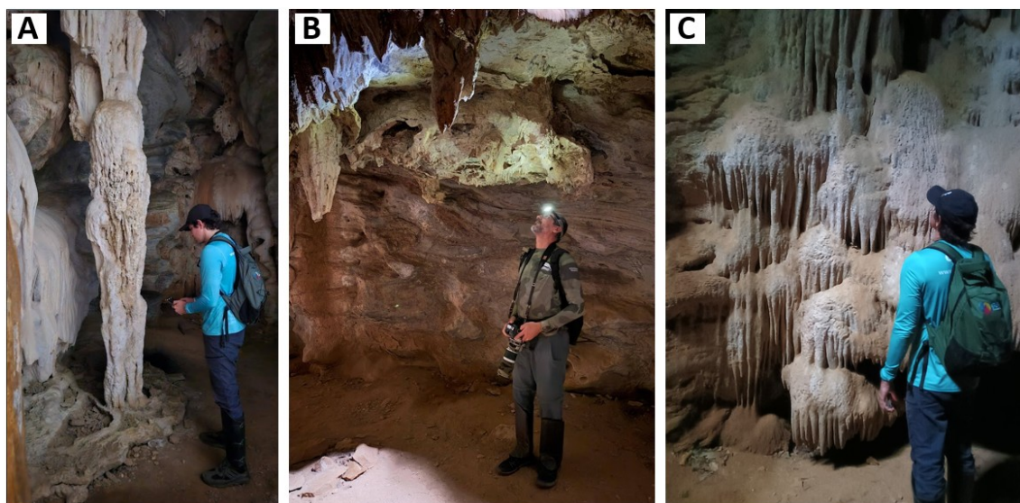
Figura 17. Espelotemas das cavernas da Furna dos Ossos. (A) Coluna; (B) Estalactites; e (C) Escorrimento. Fonte: Equipe técnica do projeto.
