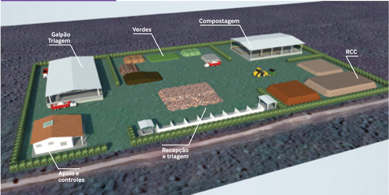
Figura I – Layout esquemático da CMR.
