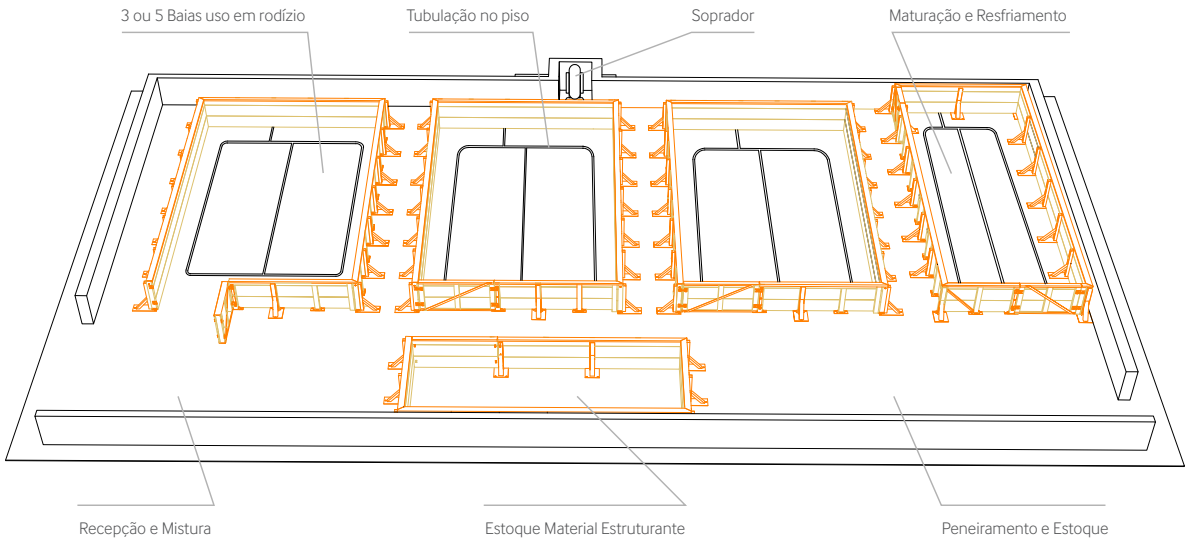
Figura 7– Desenho ilustrativo do Galpão de Compostagem .
