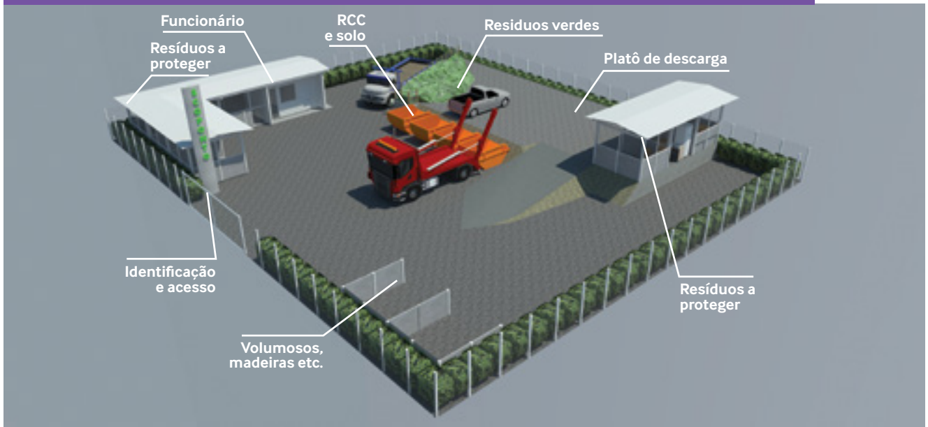
Figura 2 – Layout esquemático do Ecoponto – área em torno de 835m² para municípios onde há operação de caminhão poliguidaste.
