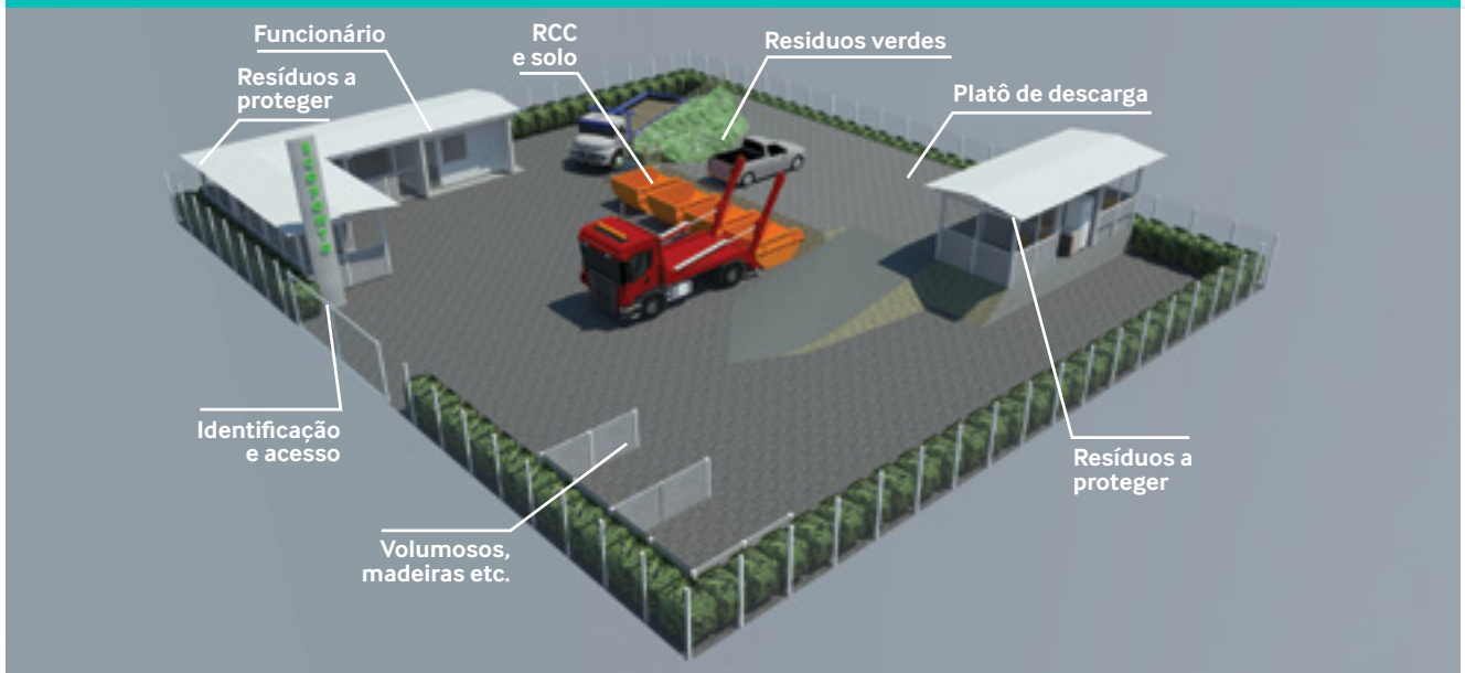
Figura 2 – Layout esquemático do Ecoponto – área em torno de 835m² para municípios onde há operação de caminhão poliguindaste.
