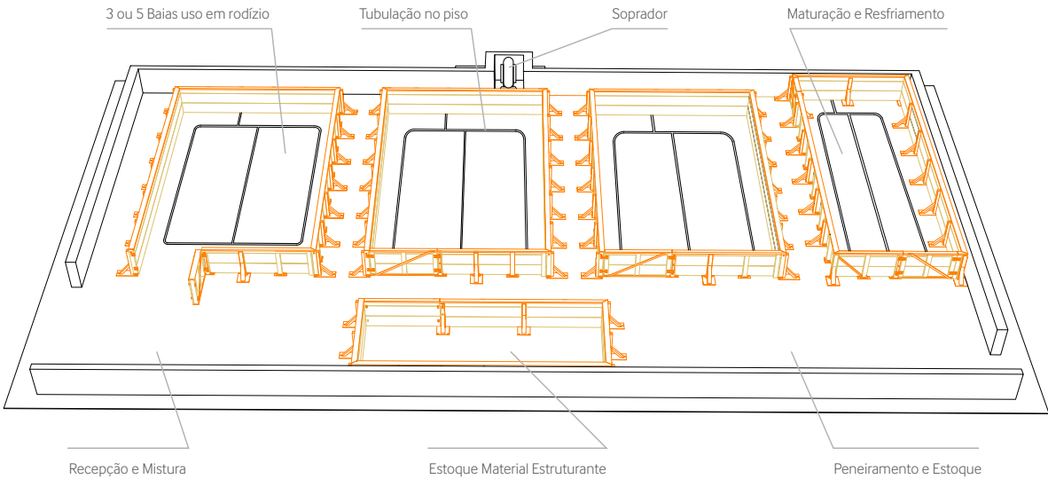
Figura 8– Desenho ilustrativo do Galpão de Compostagem .
