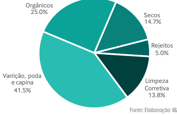
Gráfico 4 – Distribuição de despesas nos custos dos serviços de manejo de resíduos sólidos e limpeza urbana – estimativa para o Litoral Oeste.
