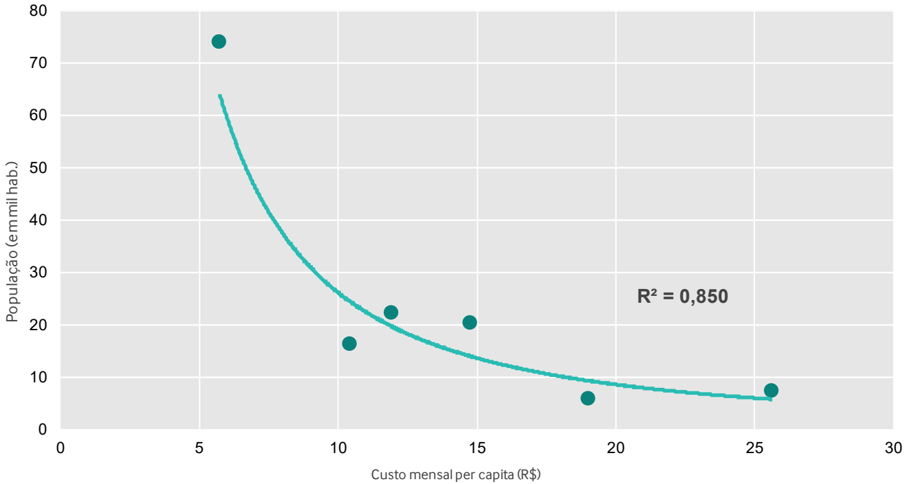
Gráfico 5 – Despesa (parcial) mensal per capita com serviços de manejo de resíduos sólidos e limpeza urbana no Litoral Oeste.
