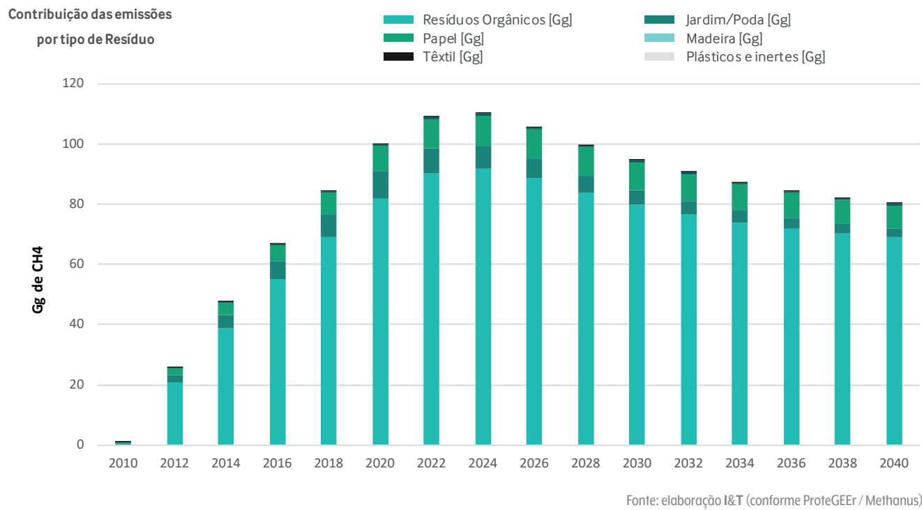
Gráfico 11 – Litoral Oeste – emissões por tipo de resíduo resultantes da alteração do seu destino (2021) com o Plano de Coletas Seletivas Múltiplas.
