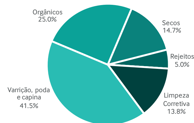
Gráfico 6 – Distribuição de despesas nos custos dos serviços de manejo de resíduos sólidos e limpeza urbana – estimativa para o Litoral Oeste.
