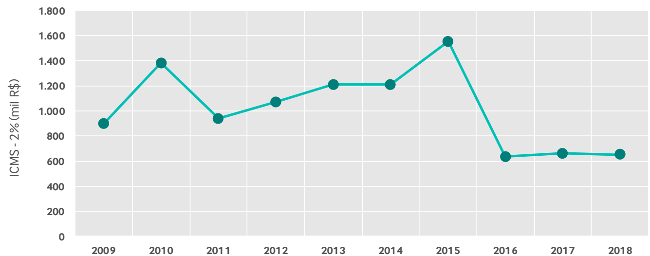
Gráfico 12 – Repasses do ICMS Sócio Ambiental na Região Litoral Oeste.
