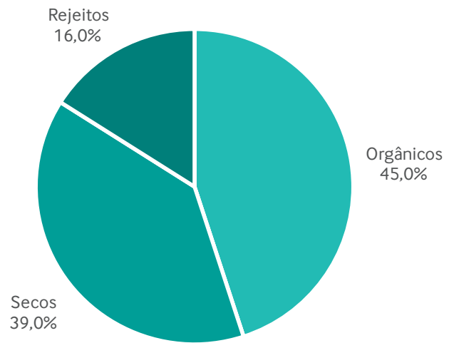
Gráfico 2 – Composição gravimétrica do Litoral Oeste.
