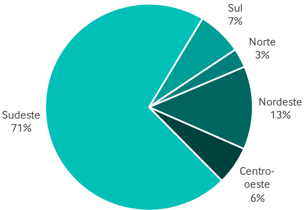
Gráfico 3 – Postos de entrega de pilhas e baterias segundo macrorregiões (%).
