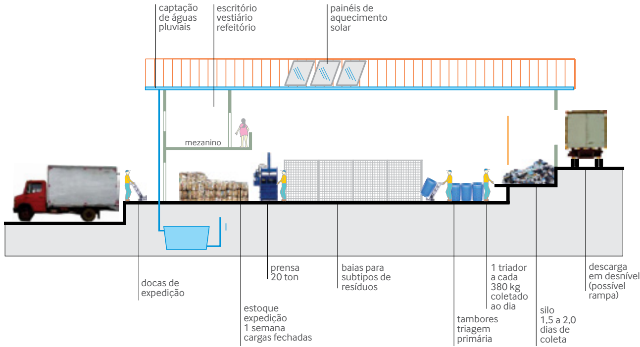
Figura 6 – Desenho ilustrativo do Galpão de Triagem de Resíduos Secos.
