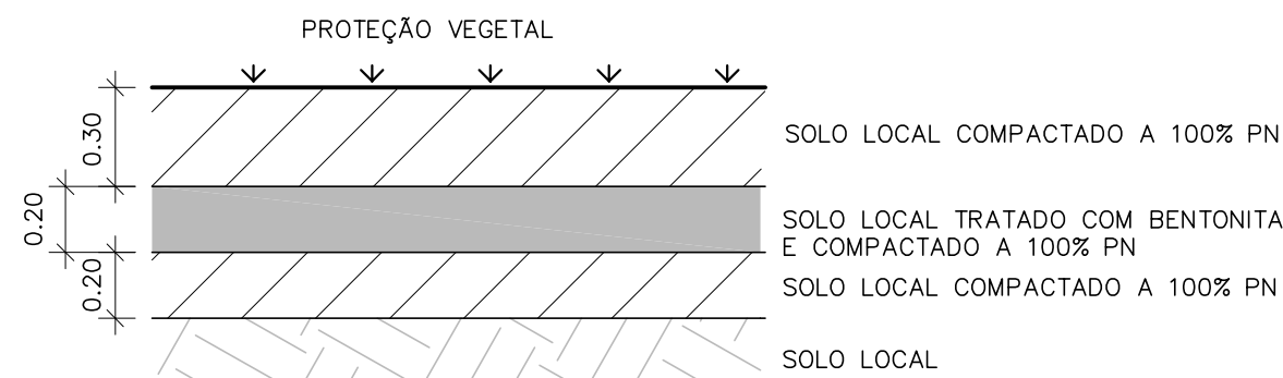
AMPLIAÇÃO C SEM ESCALA (VER NOTA 20)
