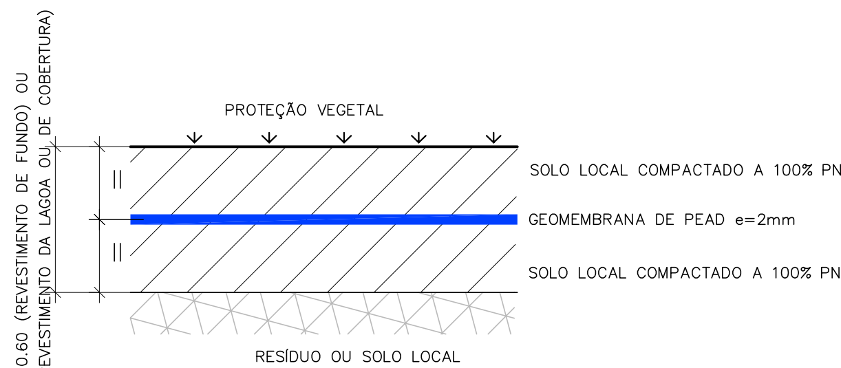
DETALHE DO REVESTIMENTO DE COBERTURA E DE FUNDO OPÇÃO COM GEOMEMBRANA DE PEAD e=2mm
