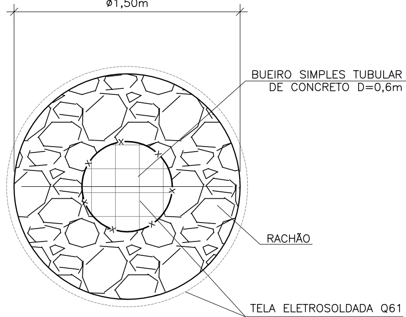
DETALHE DRENO DE GÁS SEM ESCALA (VER NOTA 15)
