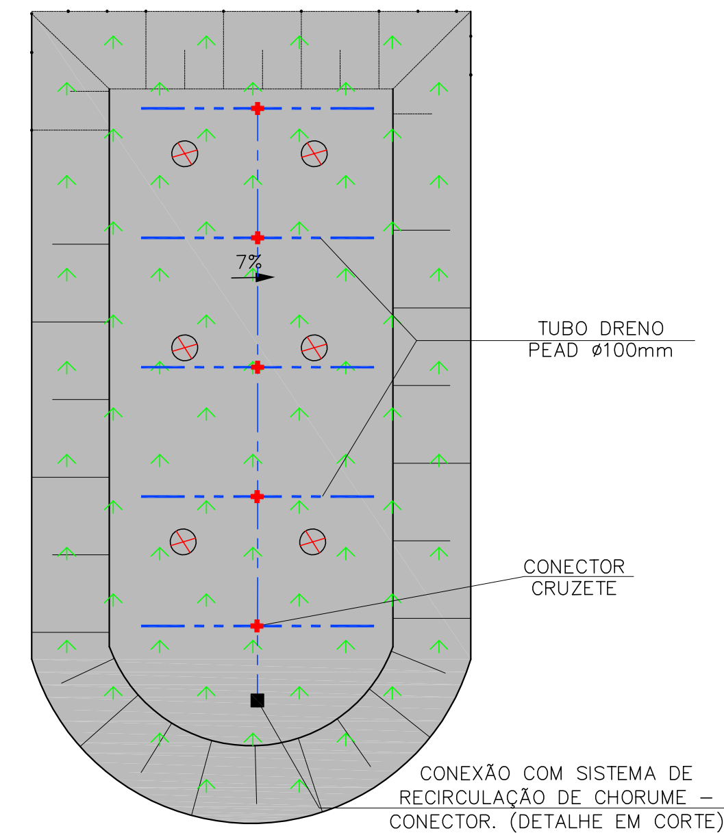
RECIRCULAÇÃO DE CHORUME SEM ESCALA
