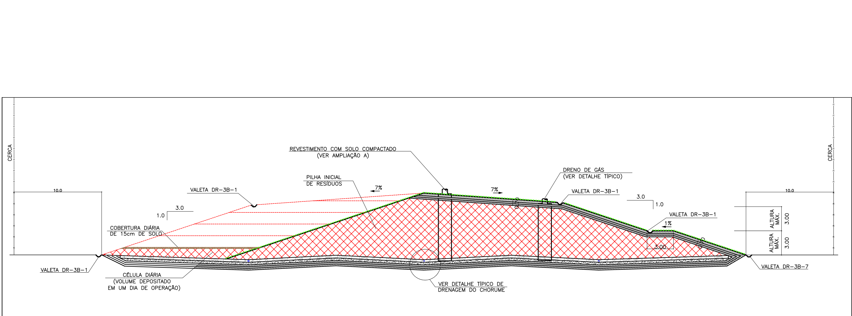
SEÇÃO A –CORTE TÍPICO SEM ESCALA
