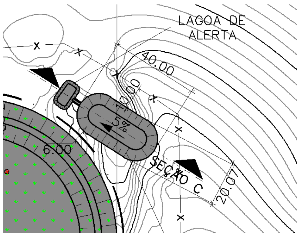
Figura 5.9 –Lagoa de chorume e lagoa de alerta do Lixão de Barbalha.
