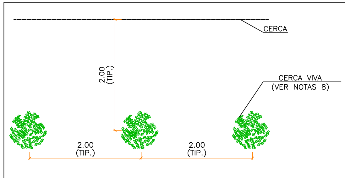
DISPOSIÇÃO CERCA VIVA SEM ESCALA
