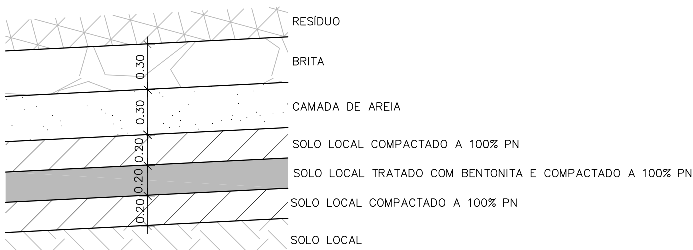
AMPLIAÇÃO B (VER NOTA 20) SEM ESCALA
