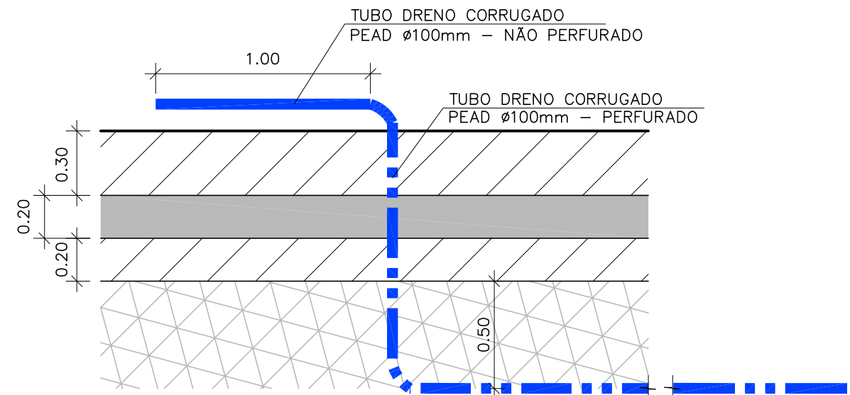
DETALHE EM CORTE SEM ESCALA
