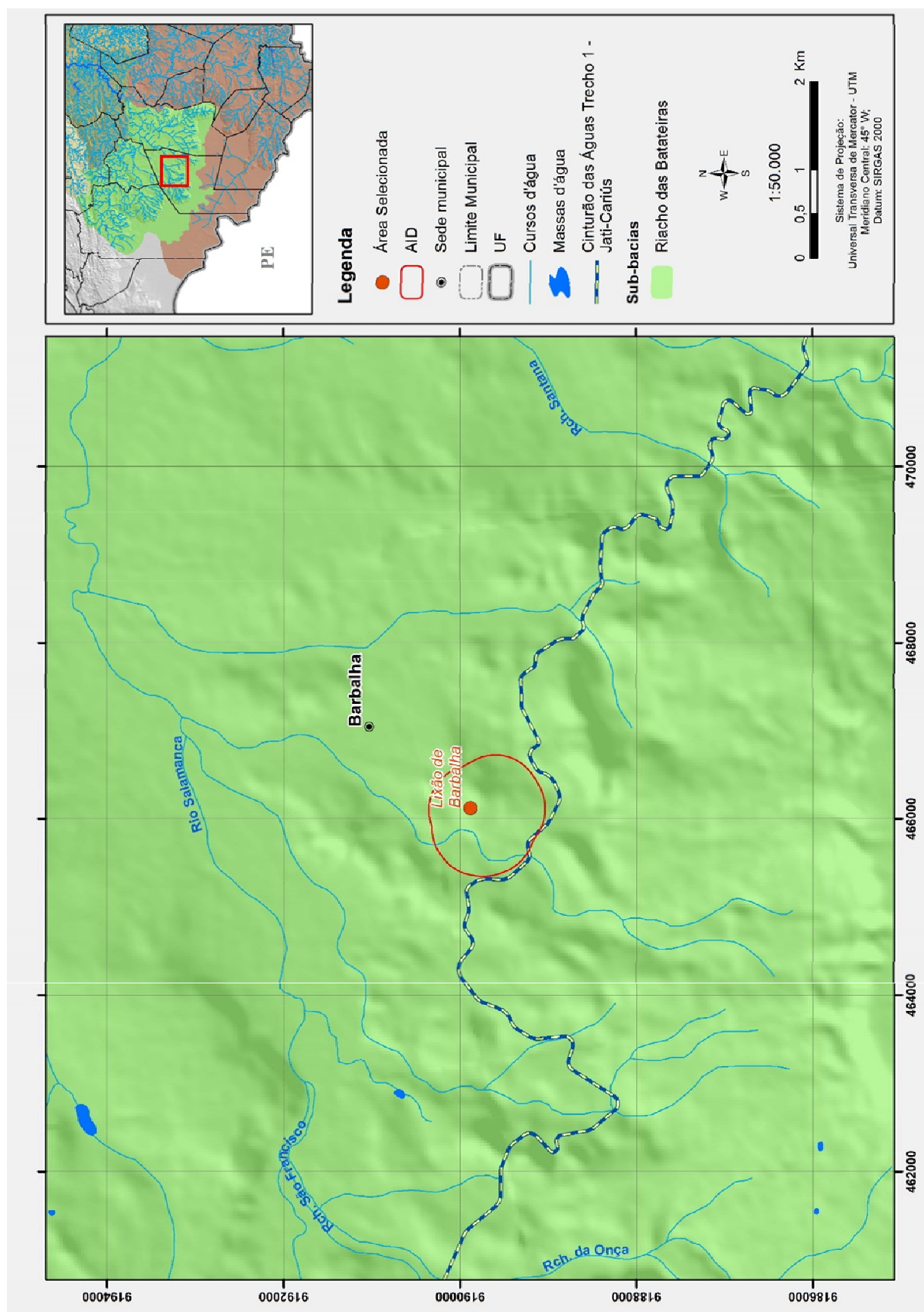
Figura 4.3 – Mapa da hidrografia na região do Lixão de Barbalha. Adaptado de FUNCEME - Fundação Cearense de Meteorologia e Recursos Hídricos - (2010). Shapefile "rios_1_100000_Salgado.shp" de 09/11/2010, enviado pela SEMA.
