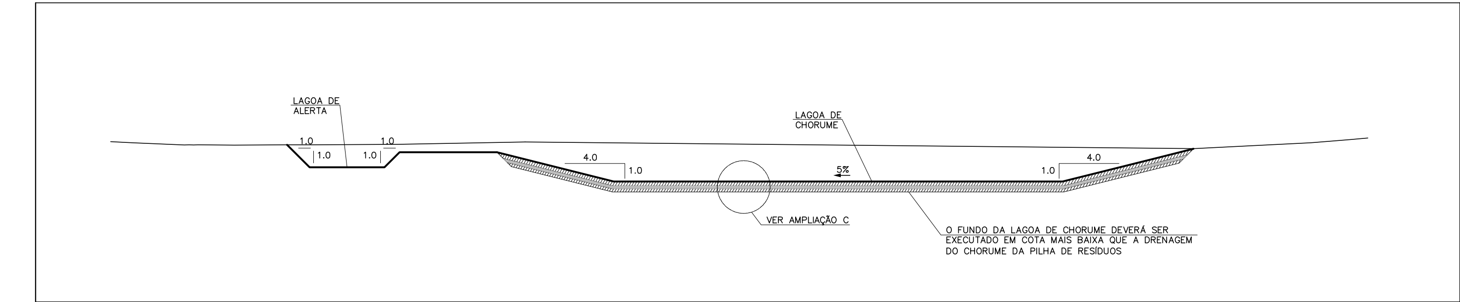
SEÇÃO B –CORTE TÍPICO SEM ESCALA
