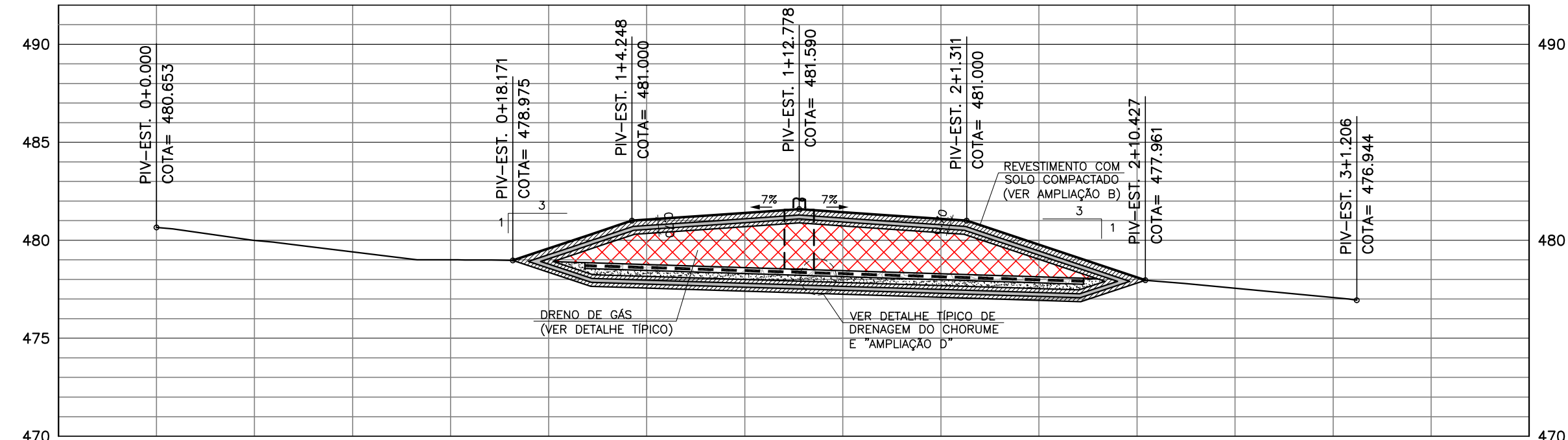
SEÇÃO 02 ESC. 1:250
