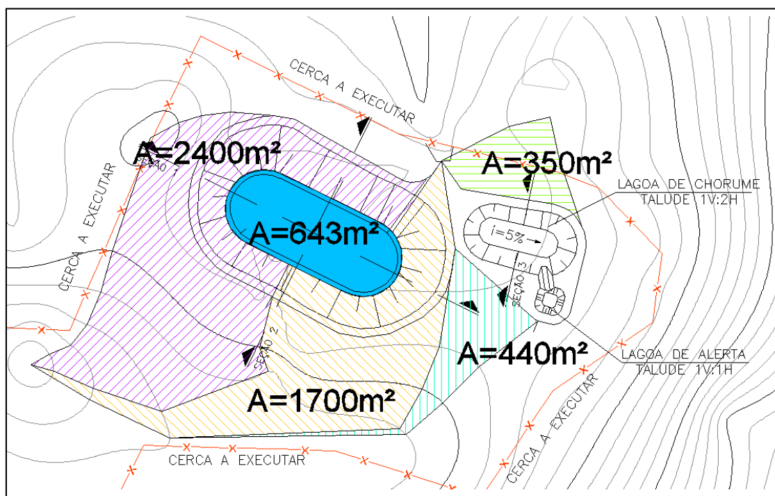
Figura 5.10 – Áreas de contribuição do sistema de drenagem.
