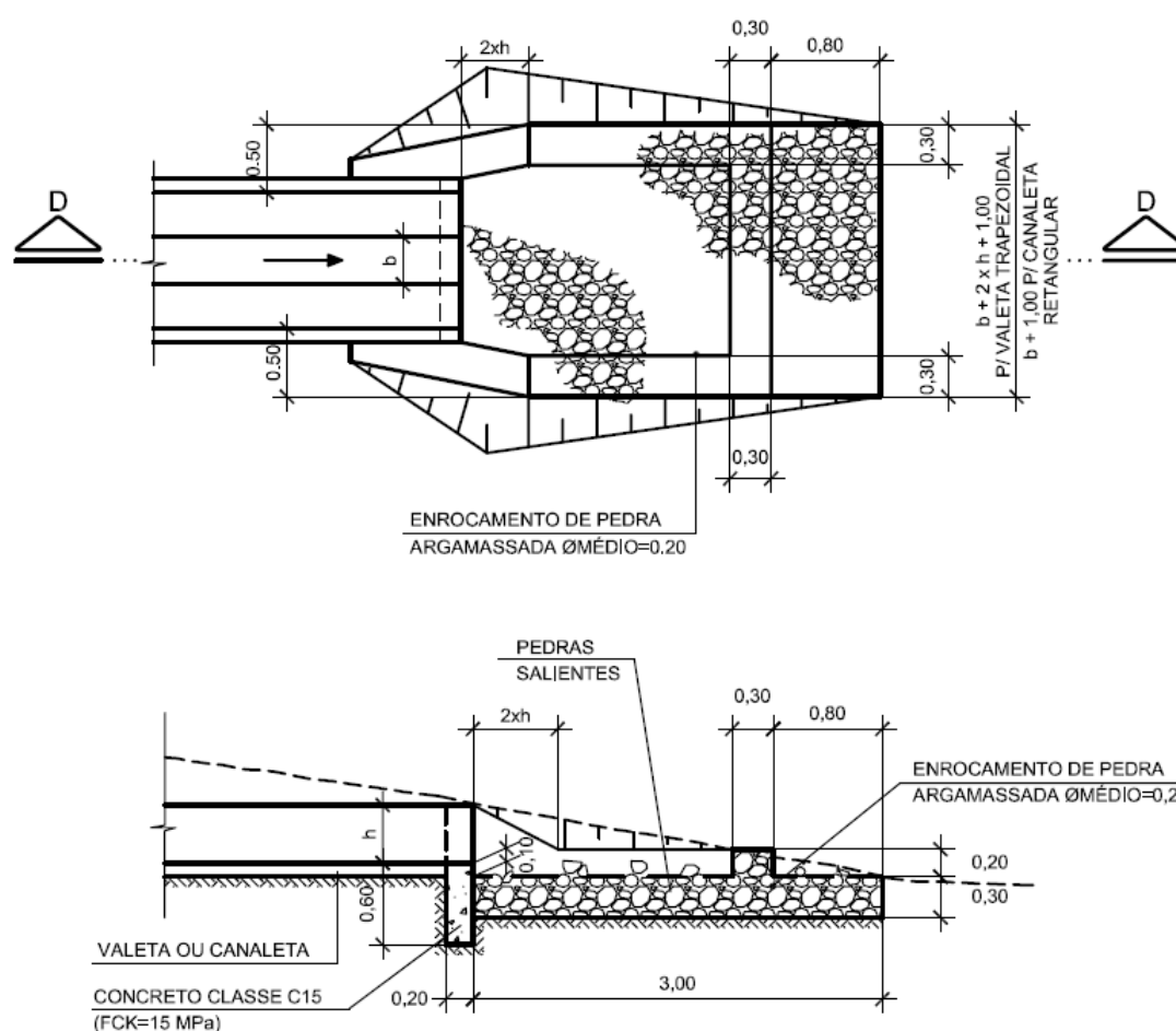
Figura 5.12 - Dispositivo de dissipação padrão DER tipo DR-10A-1.
