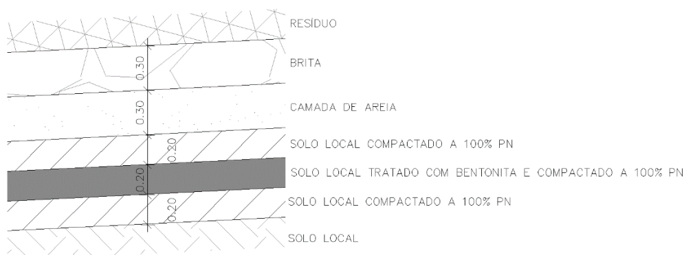
Figura 5.3 - Detalhe das camadas do revestimento de fundo e drenagem de chorume.
