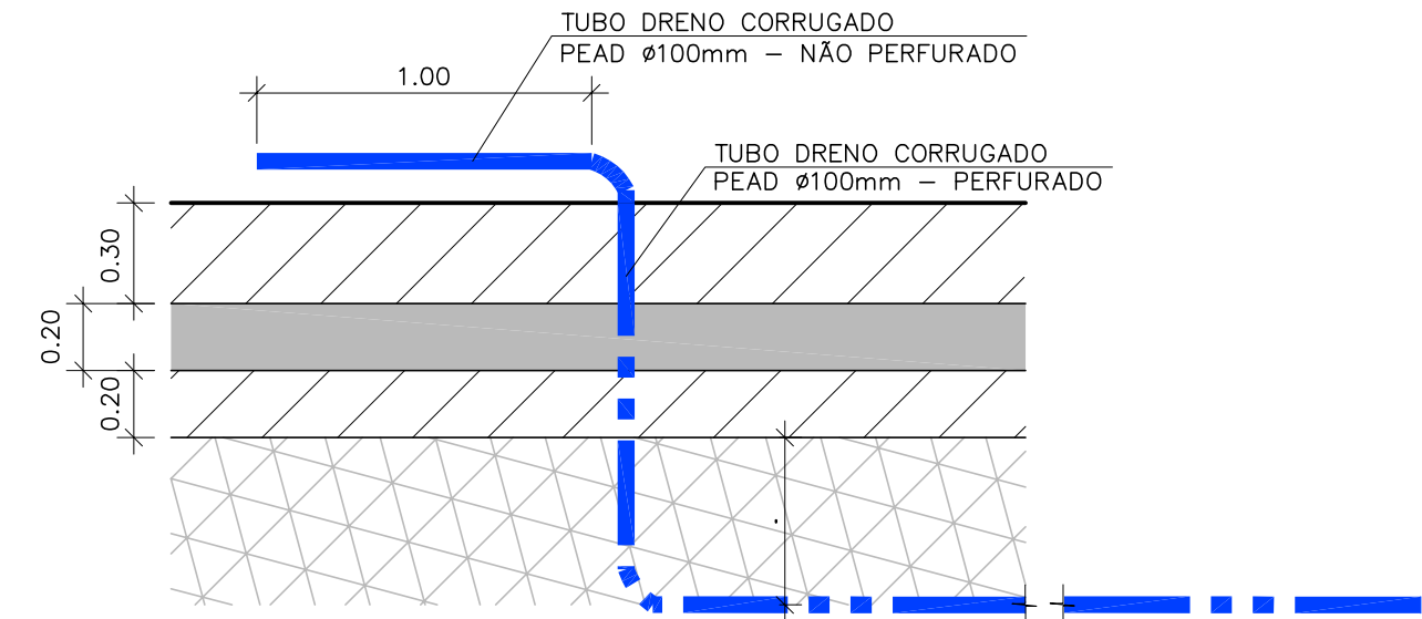
DETALHE EM CORTE SEM ESCALA
