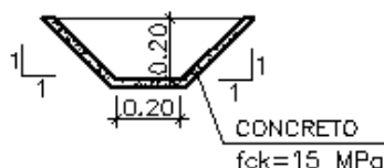
CANALETA DR-3B-1
