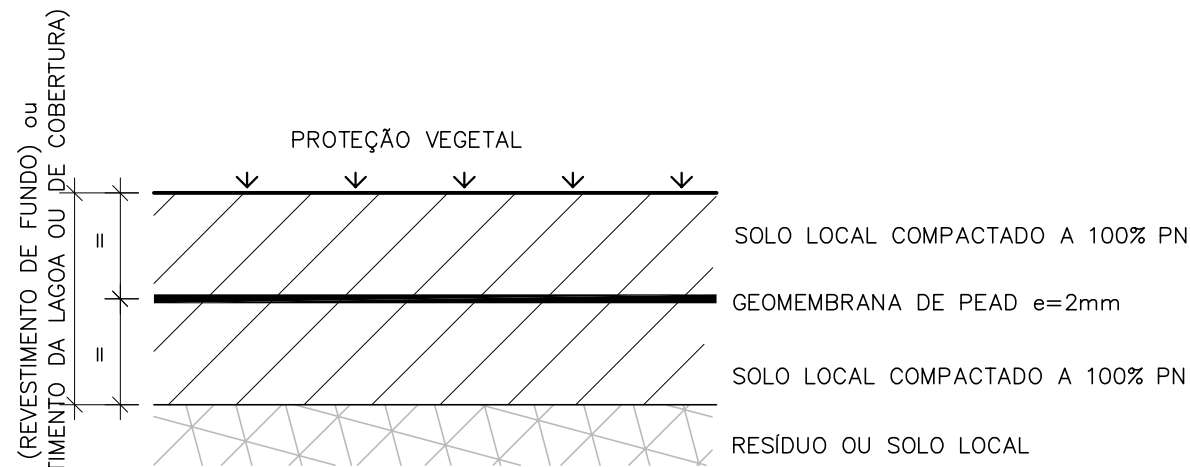
DETALHE DO REVESTIMENTO DE COBERTURA E DE FUNDO OPÇÃO COM GEOMEMBRANA DE PEAD e=2mm SEM ESCALA (VER NOTA 17)
