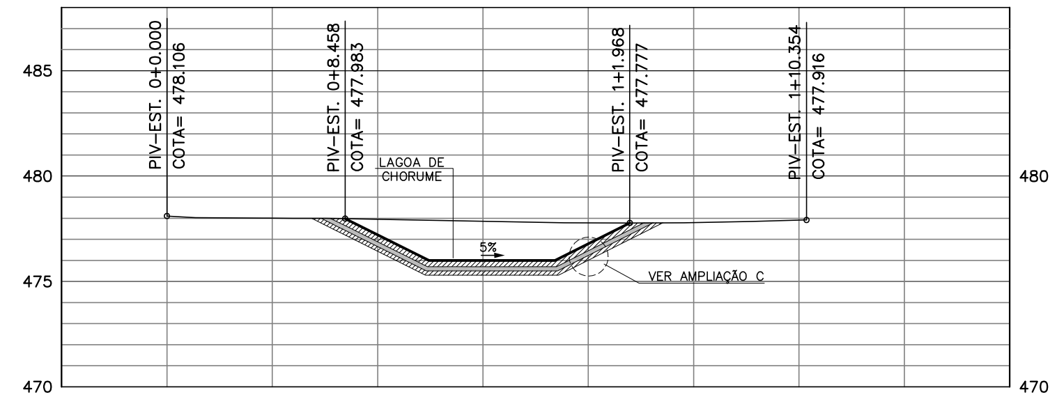
SEÇÃO 03 ESC. 1:250
