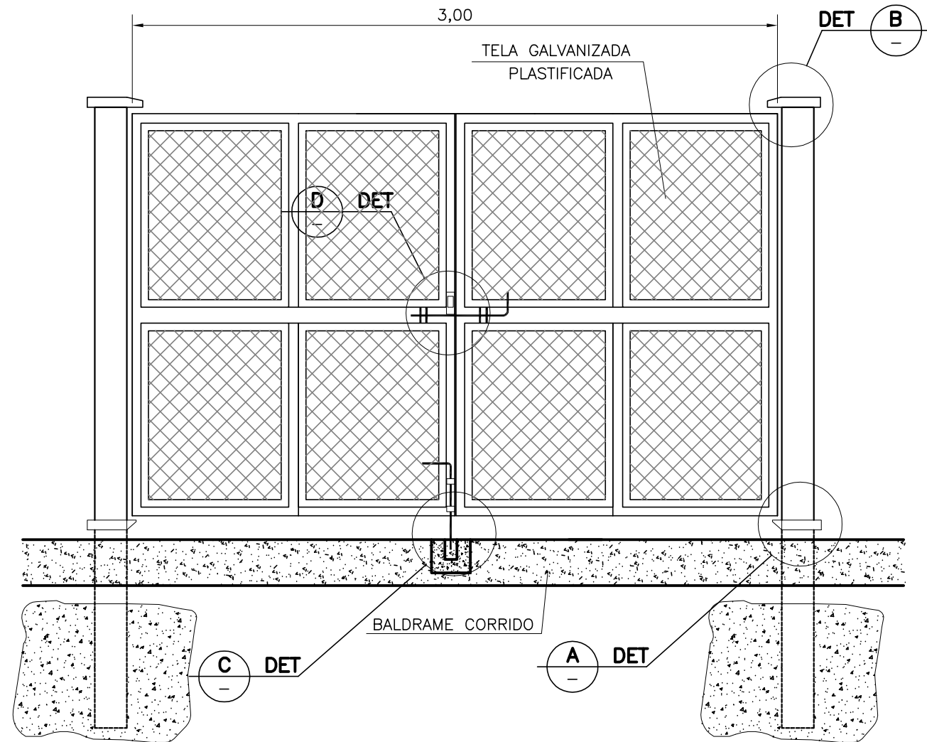
DETALHE GENÉRICO DO PORTÃO ESC.: SEM ESCALA
