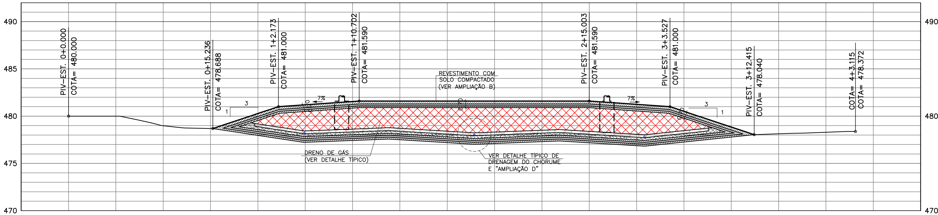
SEÇÃO 01 ESC. 1:250
