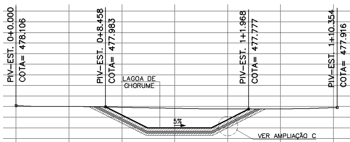
Figura 5.5 – Seção em corte da lagoa de alerta e da lagoa principal de chorume.
