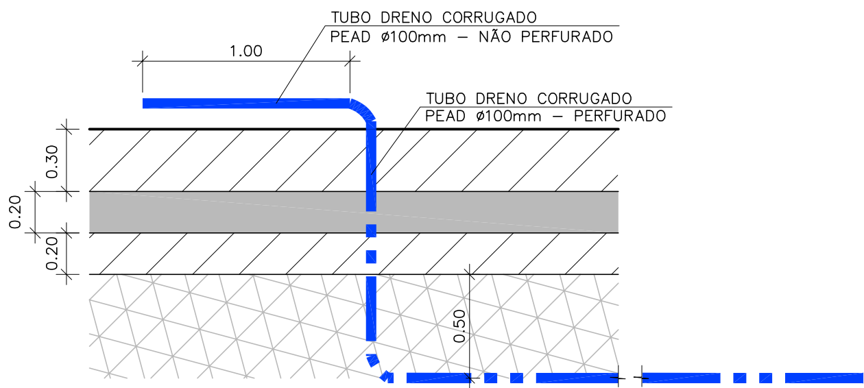
DETALHE EM CORTE SEM ESCALA
