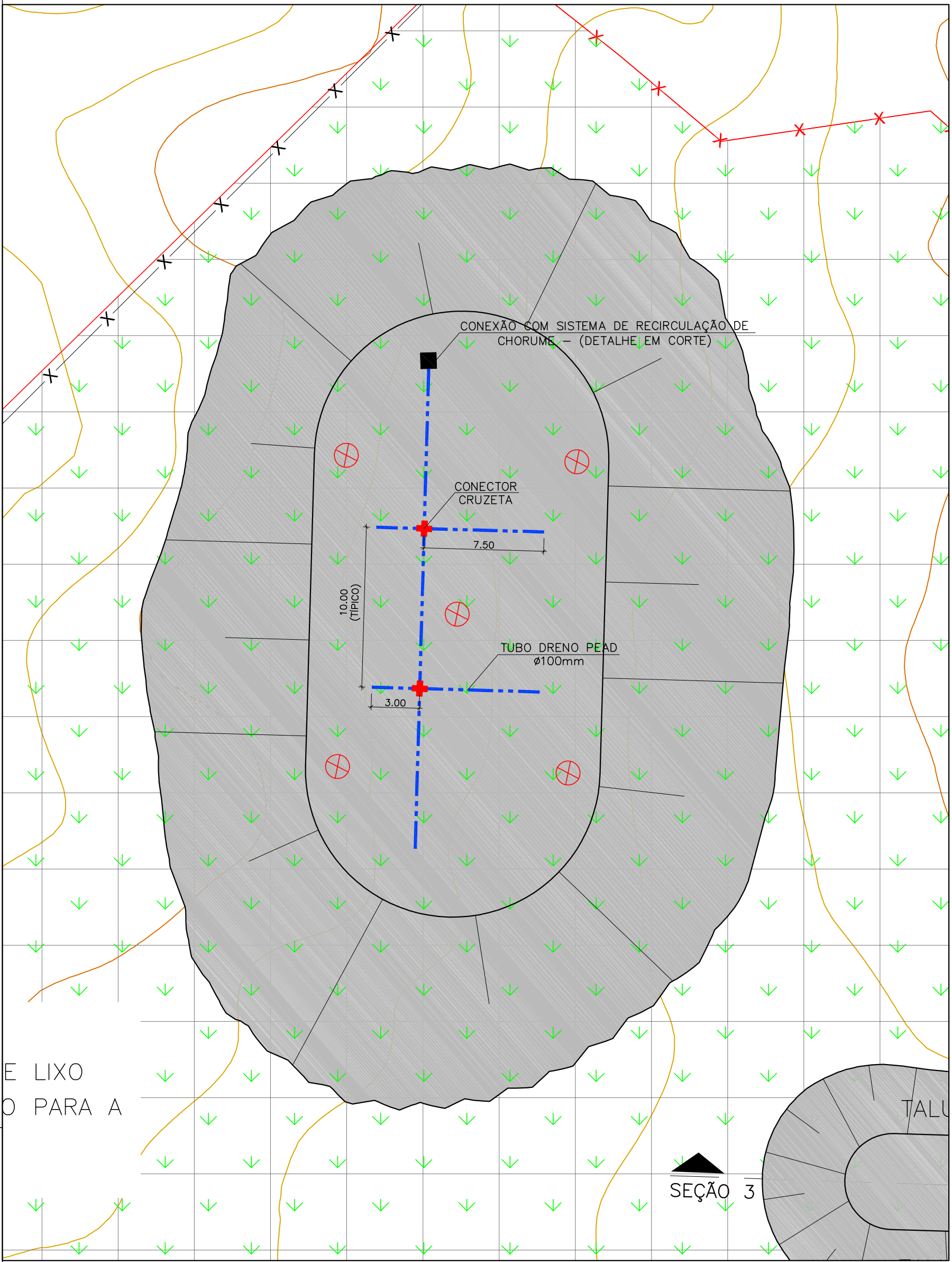
RECIRCULAÇÃO DE CHORUME ESC. 1:250
