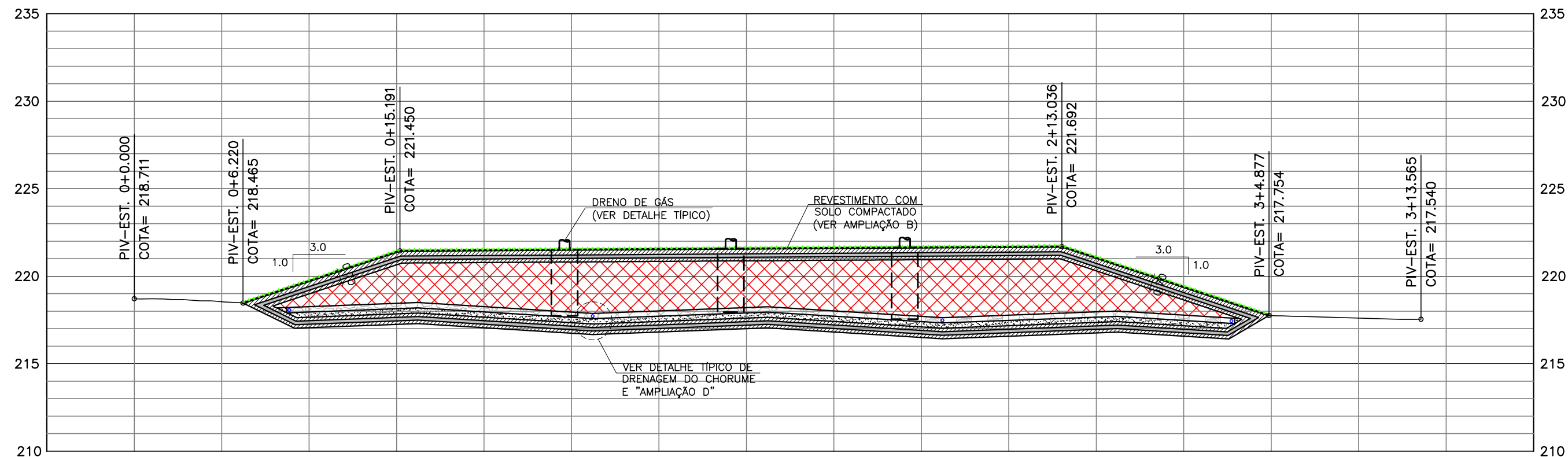
SEÇÃO 02 ESC. 1:250
