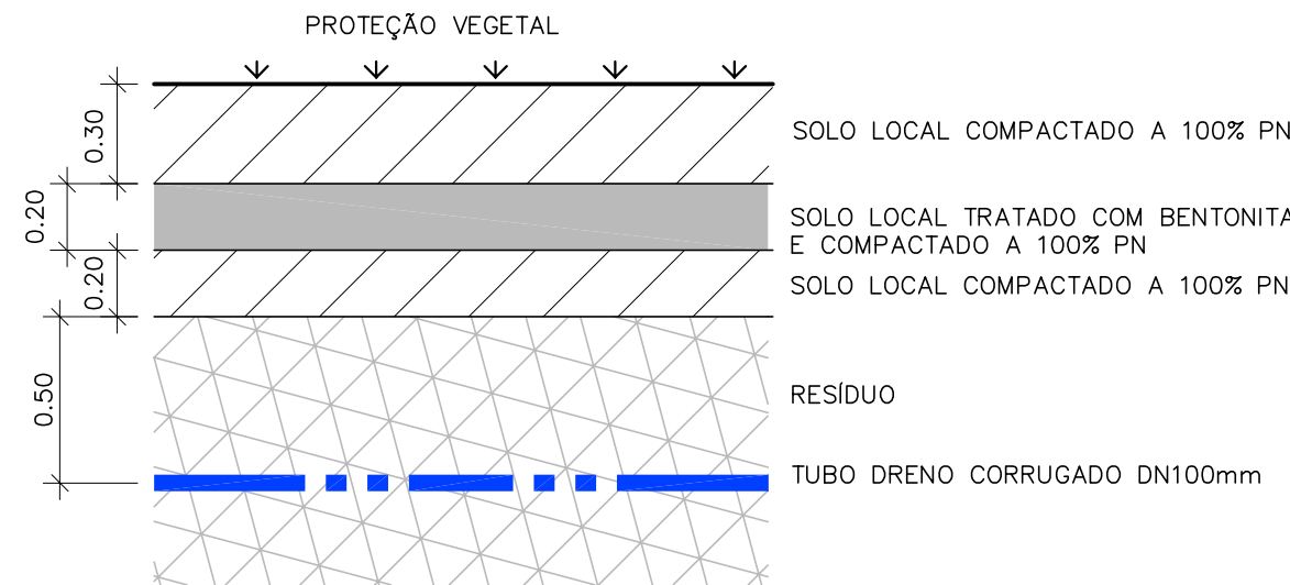
AMPLIAÇÃO B SEM ESCALA (VER NOTA 19 E 21)
