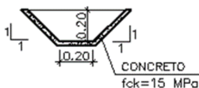
CANALETA DR-3B-1
