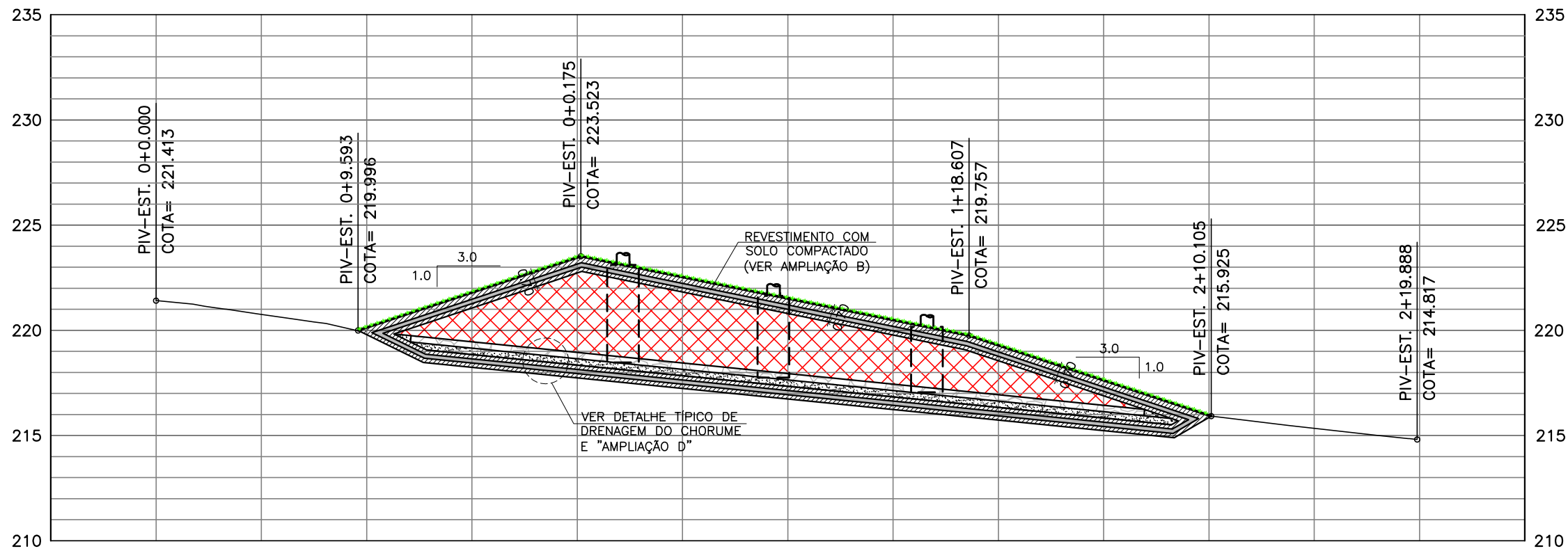
SEÇÃO 01 ESC. 1:250
