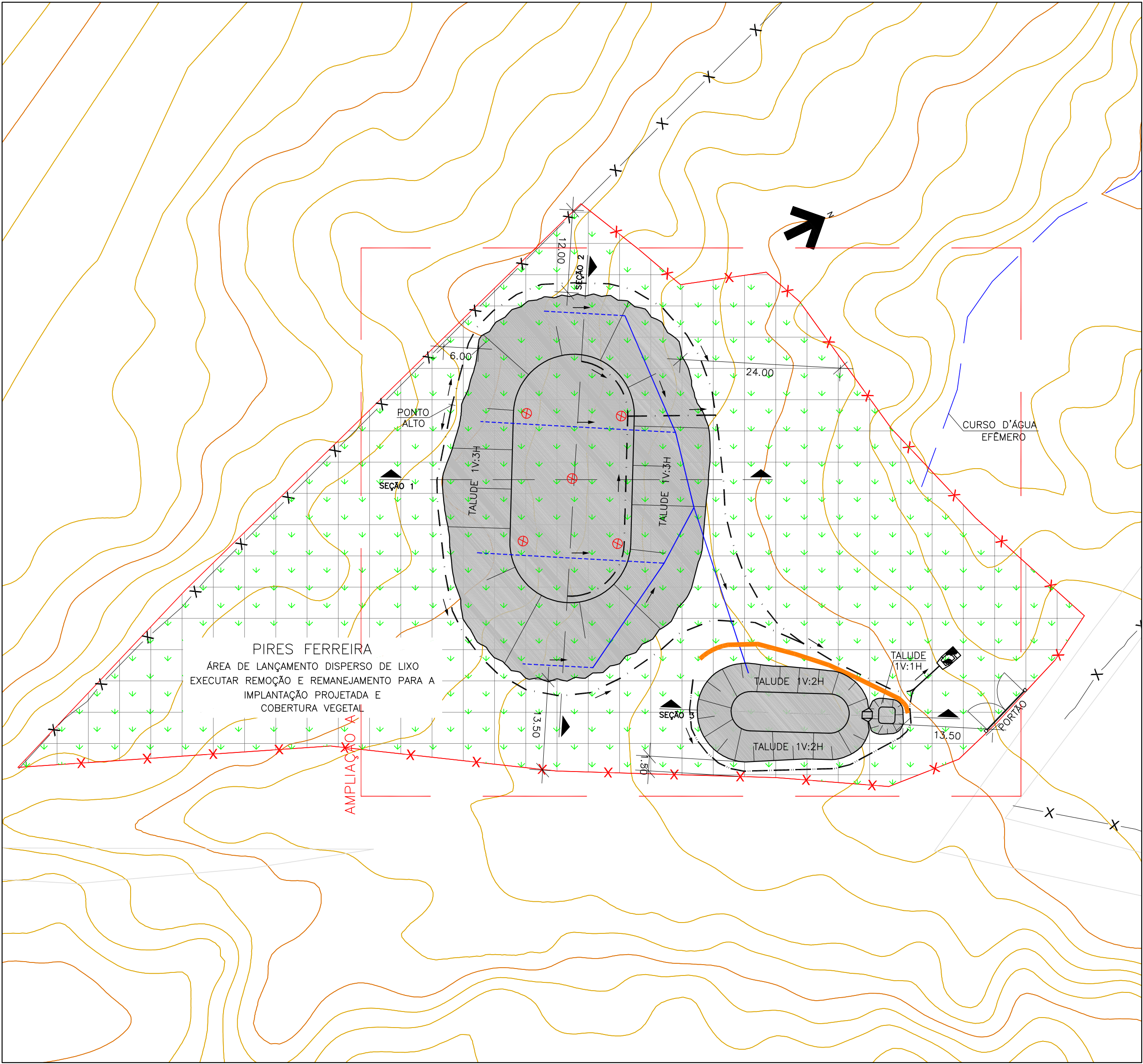
VISTA SUPERIOR ESC. 1:500
