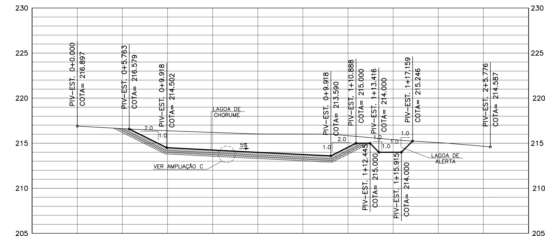
SEÇÃO 03 ESC. 1:250
