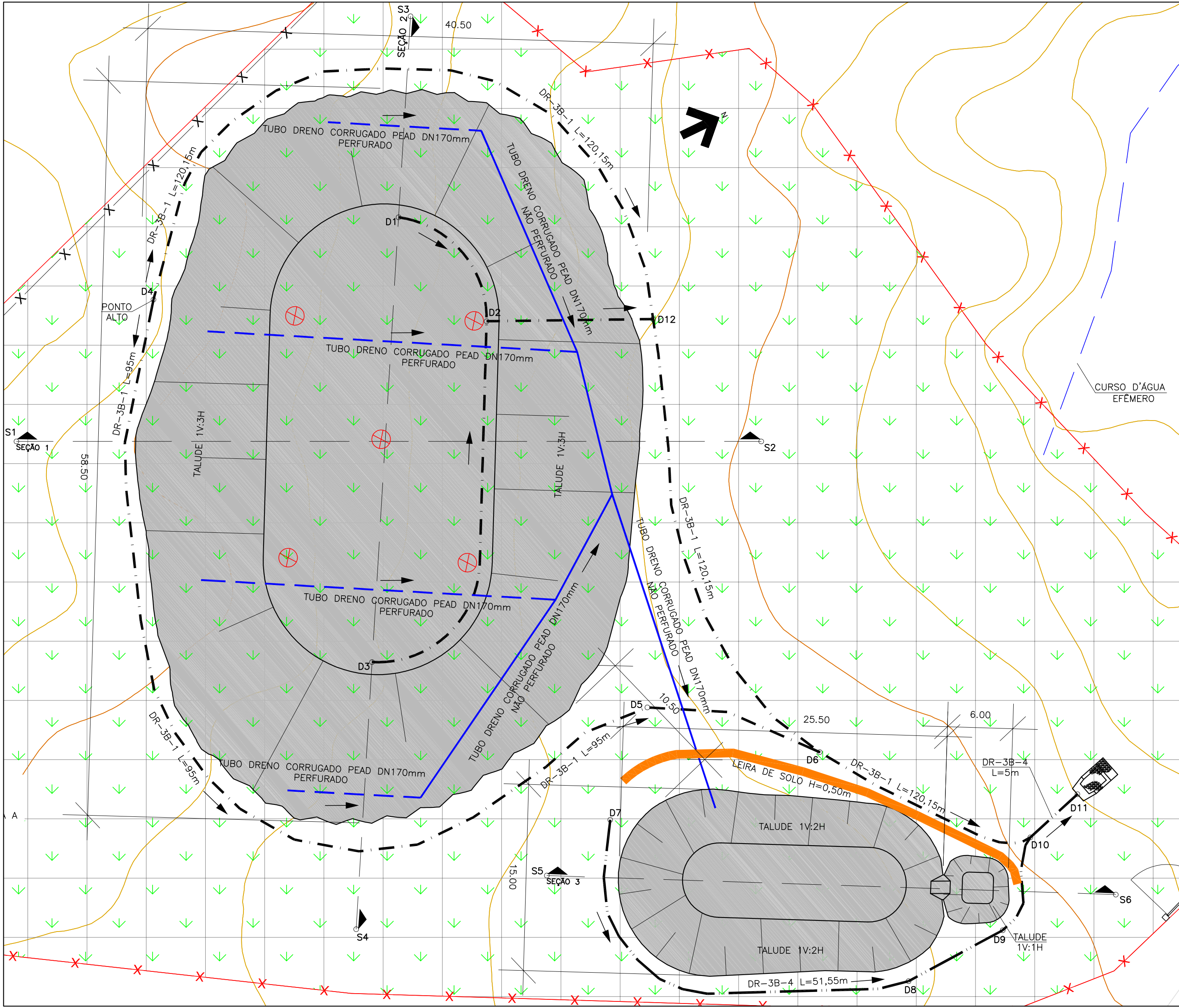
AMPLIAÇÃO A ESC. 1:250
