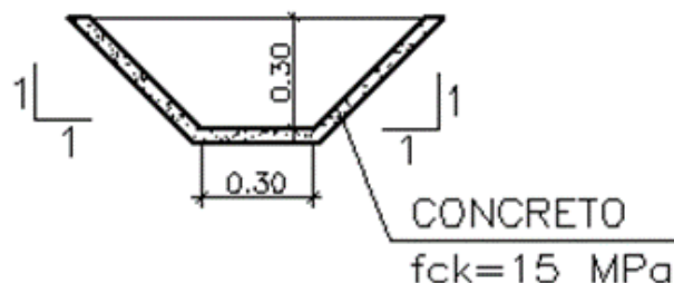
CANALETA DR-3B-4
