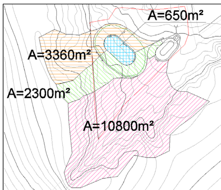
Figura 5.11 - Áreas de contribuição do sistema de drenagem.
