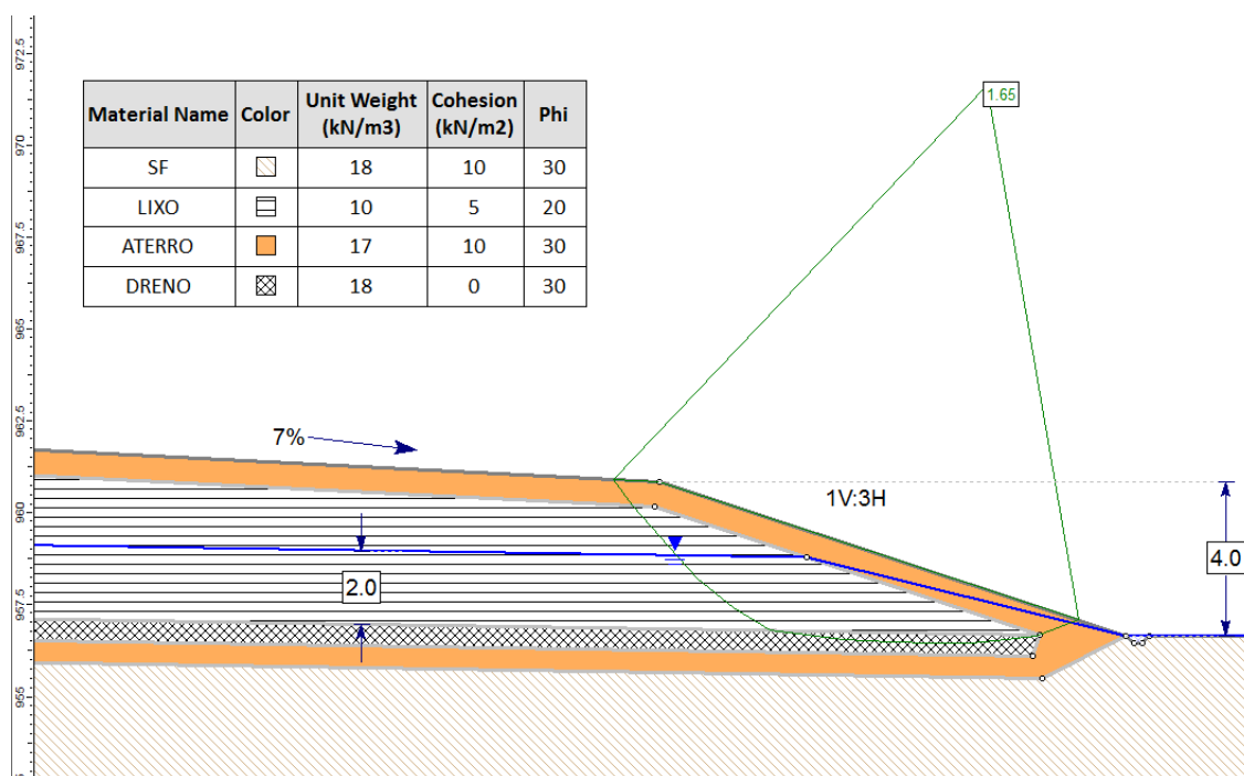
Figura 5.2 - Saída gráfica da análise de estabilidade da pilha de resíduos de Pires Ferreira. FS = 1,65.
