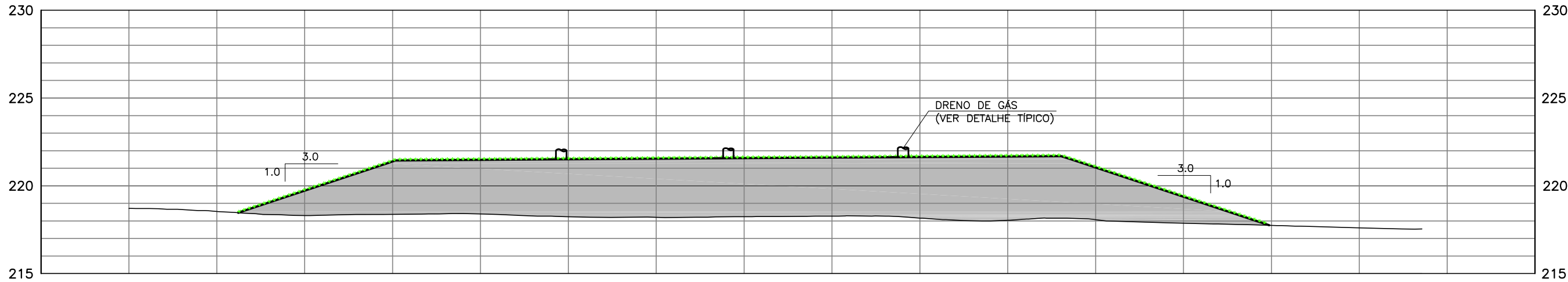
VISTA SUDOESTE ESC. 1:250
