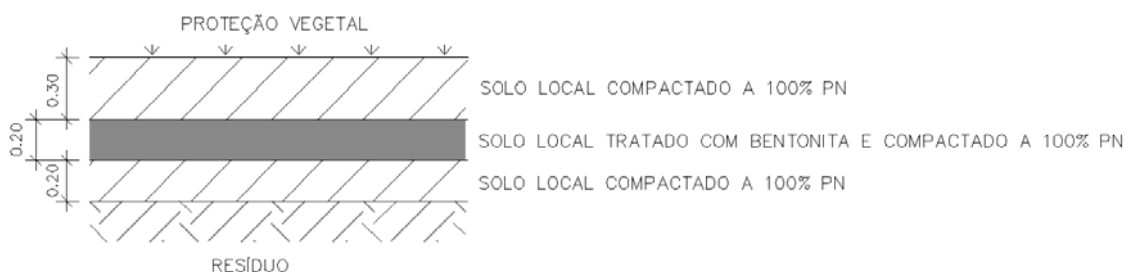
Figura 5.3 - Detalhe do revestimento de cobertura dos resíduos.
