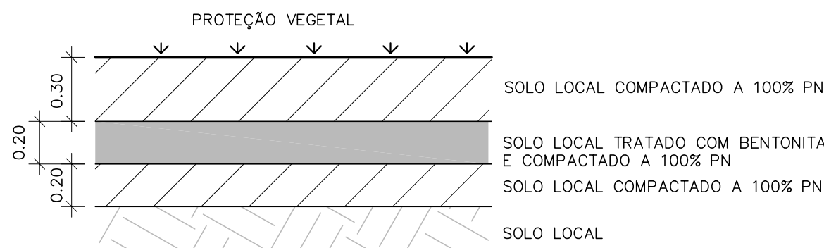
AMPLIAÇÃO C SEM ESCALA (VER NOTA 19)
