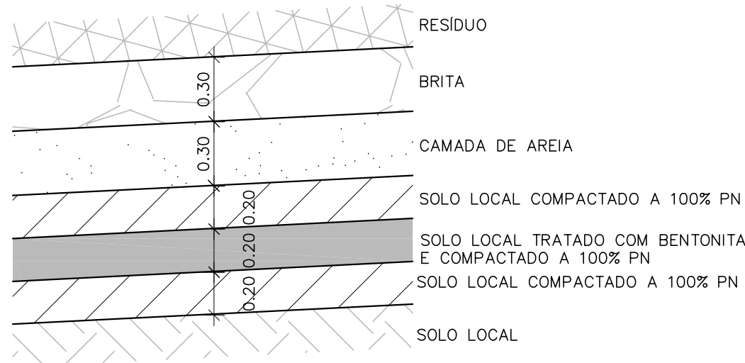
AMPLIAÇÃO D SEM ESCALA (VER NOTA 19)
