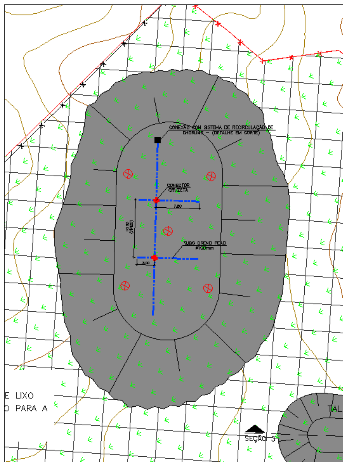
Figura 5.7 - Disposição da tubulação do sistema de recirculação de chorume.
