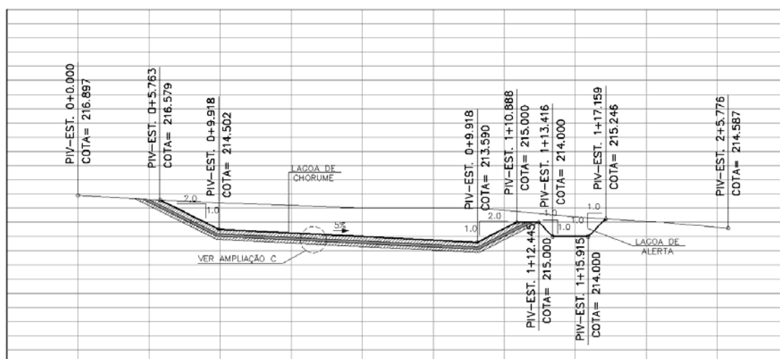
Figura 5.6 - Seção em corte da lagoa de alerta e da lagoa principal de chorume.
